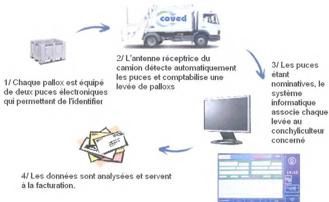
Figure 16 : Synoptique fonctionnement système de lecture des puces
