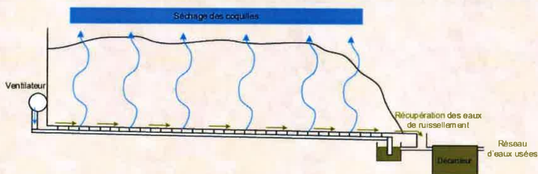
Photo 5: Illustration du fonctionnement de l'aération forcée des box d'inertage des coquilles
